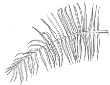
feuille pennée
