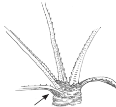
feuille palmée
