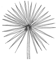
feuille palmée
