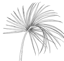
feuille costapalmée
